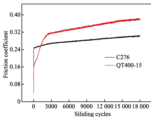
图9 熔覆层与基材摩擦系数曲线
