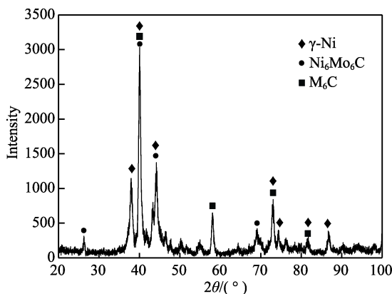
图 7 C276 熔覆层 XRD 图谱 Fig.7 XRD pattern of C276 cladding layer
