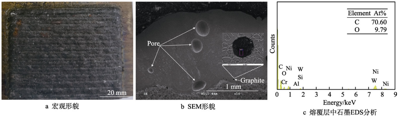
图2 熔覆层形貌
