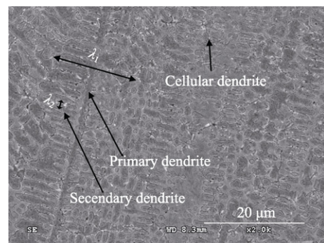
图5 熔覆层中间部位SEM形貌
