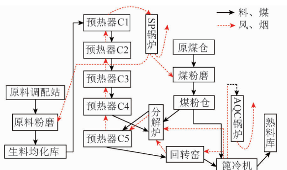
图1 新型干法水泥熟料生产线工艺流程
