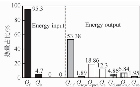
图 3 炉窑 4 个节点系统的热量收入与支出对比
