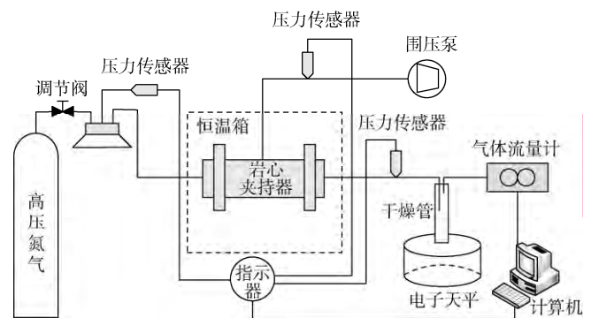
图2 非稳态法测定气水相对渗透率装置示意图
