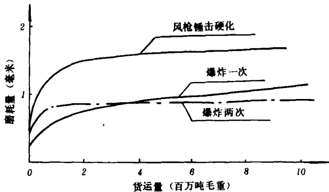
图1 磨损曲线图
