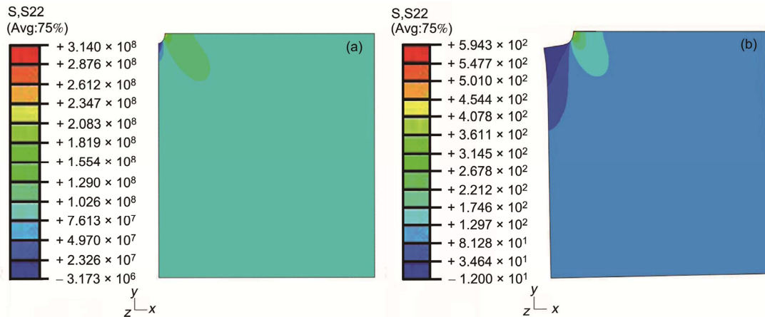
图5 (网络版彩图)缺口试样有限元计算应力云图。(a) 名义 K_t=3 ; (b) 名义 K_t=5
