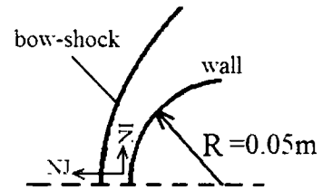
图 2 物理模型和尺寸
