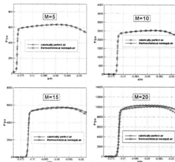
图 6 真实气体效应对流场中沿流线压力分布的影响
