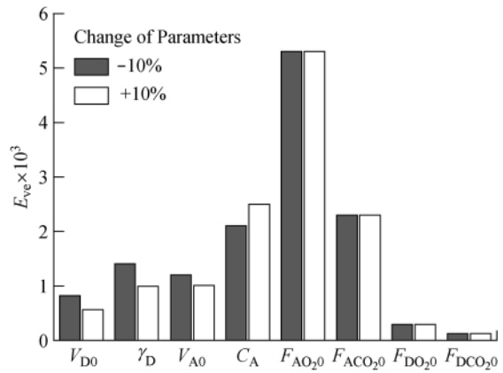
图4 参数敏感性分析
