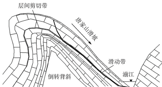
图 8 唐家山滑坡地质发育机制
