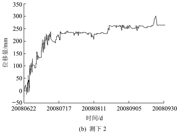
图 10 地表位移监测点时间 - 位移曲线 Fig.10 Time-displacement curve of monitoring site
