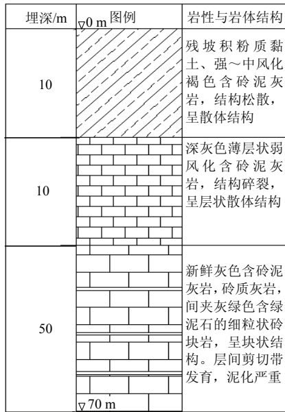
图 4 唐家山滑坡滑体结构柱状图
