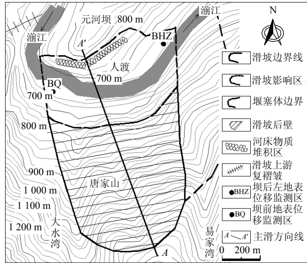
(a) 平面图
