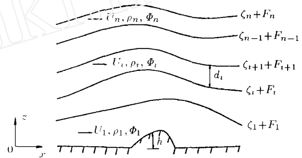
图 1 n 层流体坐标系统
