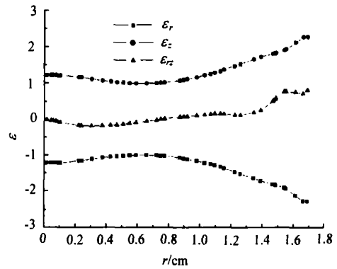
图 6 z = 4 cm 处材料横截面上的应变分布
