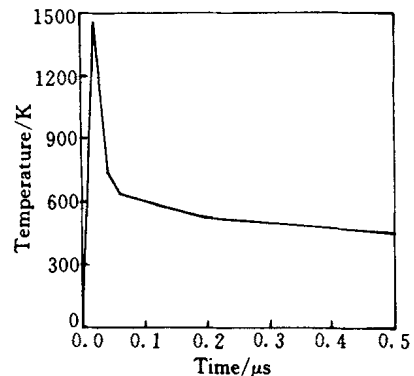
图 3 光斑中心温度的时间演化规律
