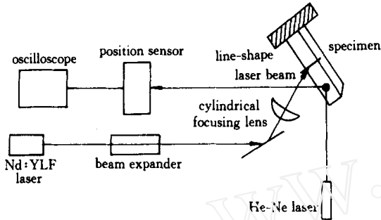
图 1 激光微弯曲加工示意图
