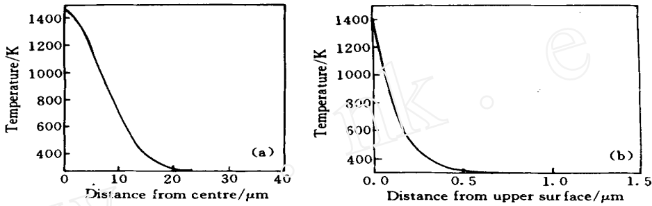
图 4 温度沿表面(a)和厚度方向(b)的分布规律
