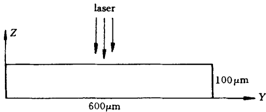
图 2 计算模型图
