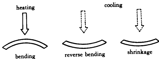
图 7 微尺度弯曲的基本过程
