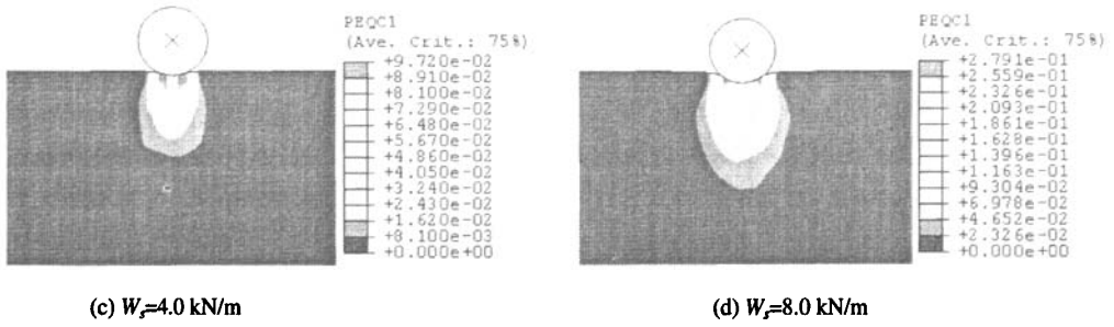
图 4 不同水下重量管道下方的土体塑性变形区( D=0.5\text{m} )
