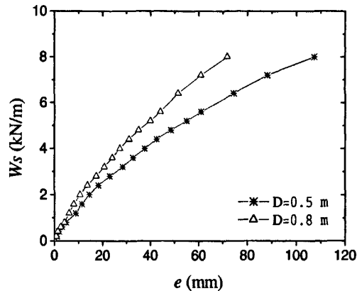
图 10 不同管道直径情况下管道沉降量与管道水下重量之间的关系
