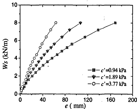
图9 不同土体粘聚力情况下管道沉降量与管道水下重量之间的关系(D=0.5m)
