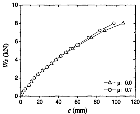
图 11 不同管土摩擦系数情况下管道沉降量与管道水下重量之间的关系 ( D=0.5\text{m} )
