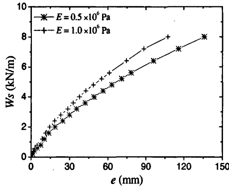
图 5 两种弹性模量情况下海底管道的沉降量与管道水下重量的关系( D=0.5\text{m} )
