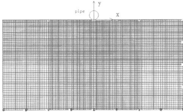
图1 有限元模型
