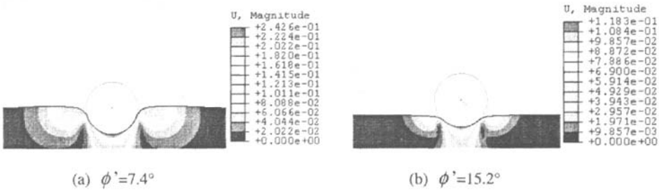
图8 不同土体内摩擦角情况下管道附近土体的位移云图(D=0.5m)
