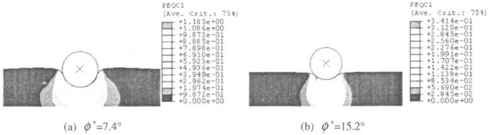
图7 不同土体内摩擦角时管道附近土体的塑性应变云图(D=0.5m)
