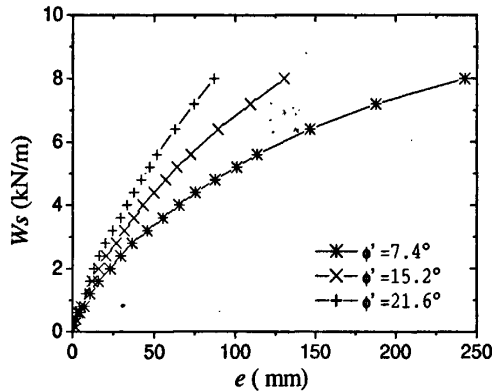
图 6 不同土体内摩擦角情况下海底管道的沉降量与管道水下重量的关系( D=0.5\text{m} )
